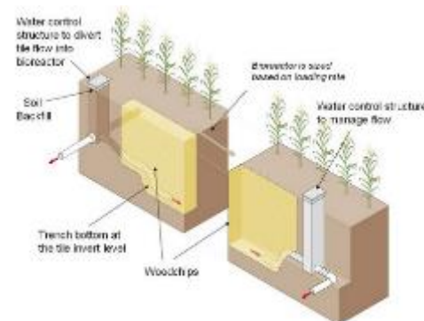
Bioreactor
